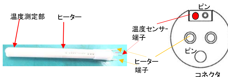
ヒーターの接続
